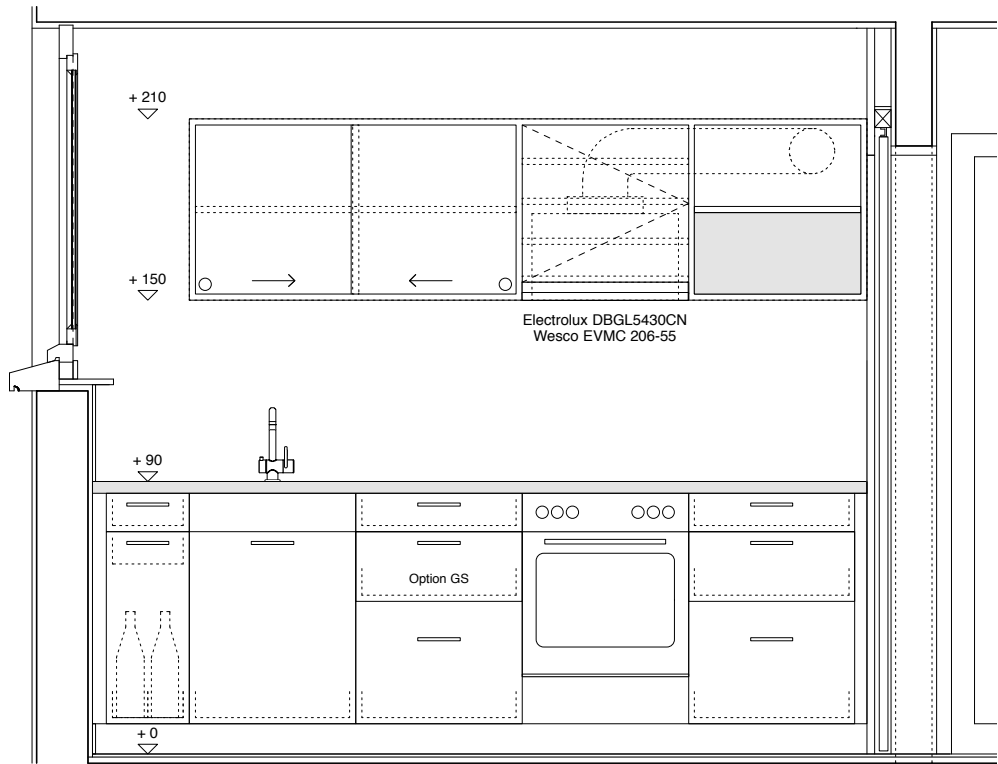
A - A Untersch. 275 x 762 x 555 mm Element mit einer 1/6-Schubl. und 5/6-Flaschenauszug Unterschrank 550 x 762 x 555 mm Kehrichtelement mit Auszug 550 x 762 x 460 mm Option GS Unterschrank 550 x 762 x 555 mm Element mit je einer 1/6-, 2/6- und 3/6-Schublade Unterschrank 550 x 762 x 460 mm für Einbau Herd V-Zug Comhair S, Front weiss Unterschrank 550 x 762 x 555 mm Element mit je einer 1/6-, 2/6- und 3/6-Schublade
